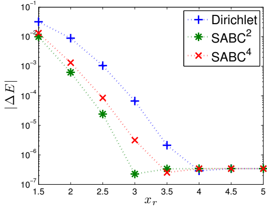
(a) Eigenvalue
