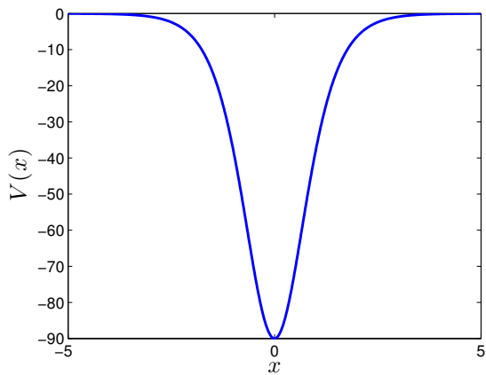
(a) Pöschl-Teller potential
