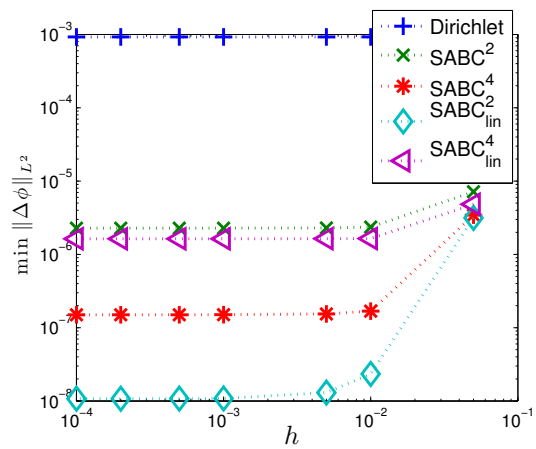
(b) Eigenfunction
