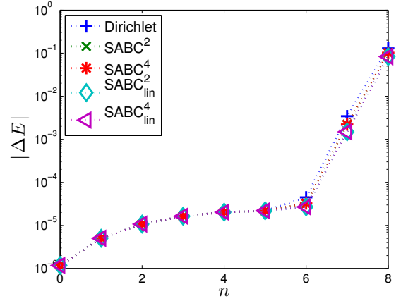
(d) x_r = 4 (direct)
