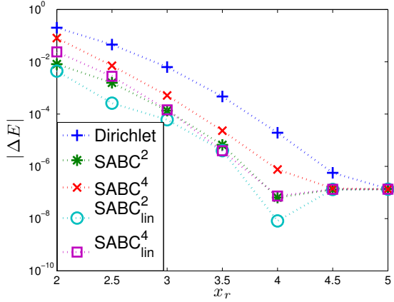
(a) Eigenvalue
