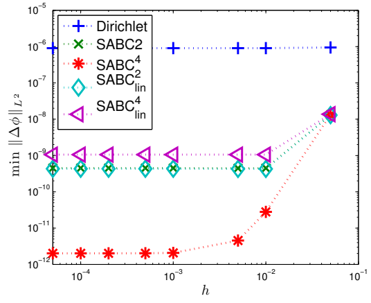
(b) Eigenfunction
