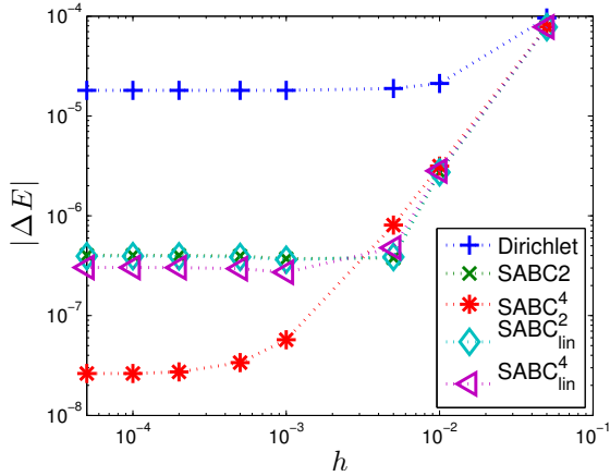
(a) Eigenvalue
