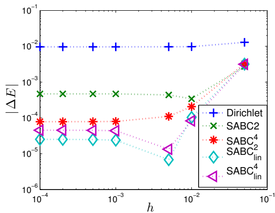
(a) Eigenvalue
