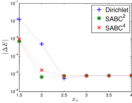
(a) Eigenvalue
